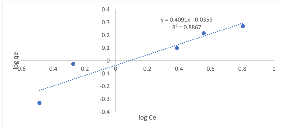
Fig. 15. Freundlich for Cd on MHFS
