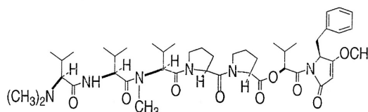
Fig. 3. Dolastatin 15 [44]
